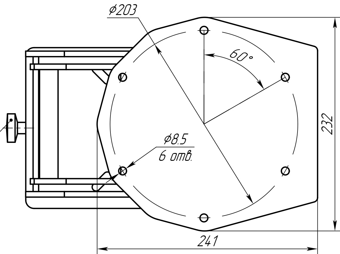
Регулятор жёсткости амортизатора
